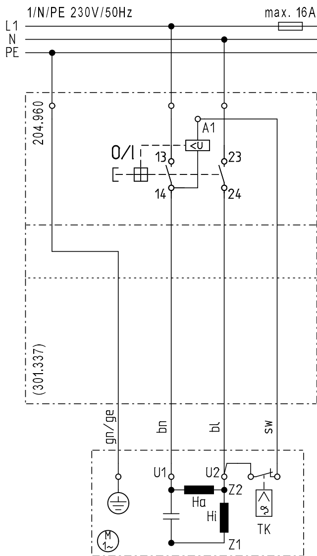
Motorschalter/motor switch 204.960 (und/and Zubehör/Option 301.337)
