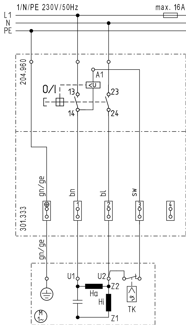
Motorschalter/motor switch 204.960 und/and Zubehör/Option 301.333
