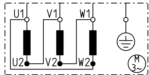
Dreieckschaltung
