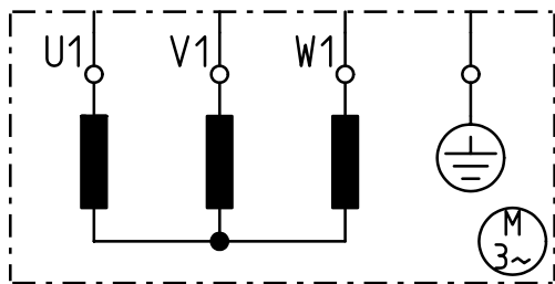
Sternschaltung
